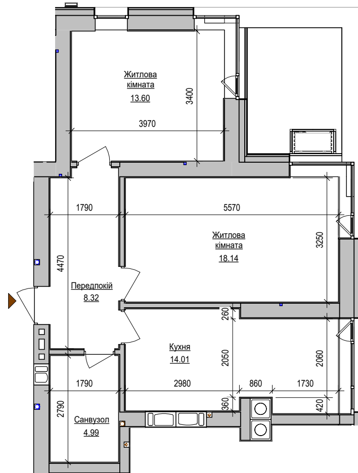
План із розмірами
