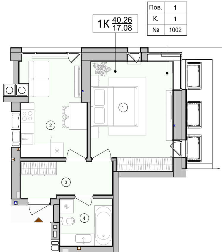
План із меблями
